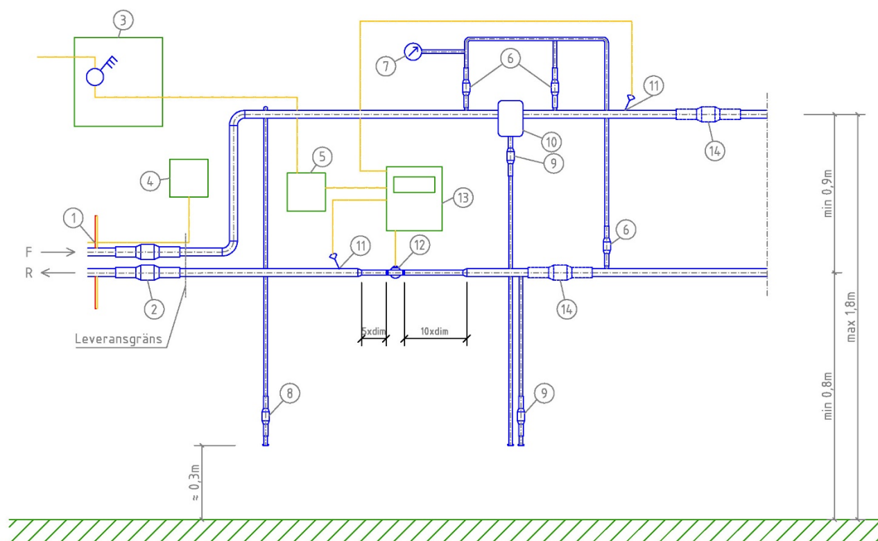
Bild 2 Principschema på mätarplats
