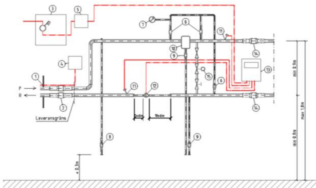
Bild 2 Principschema på mätarplats
